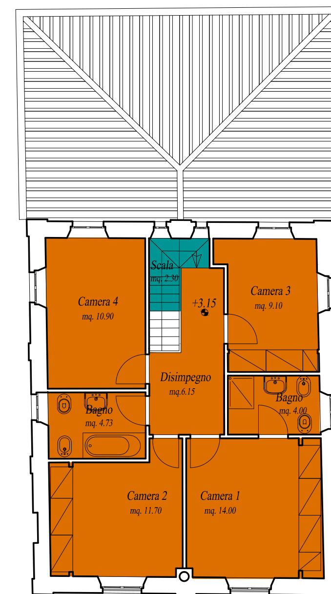
EX-STALLA PIANO PRIMO
