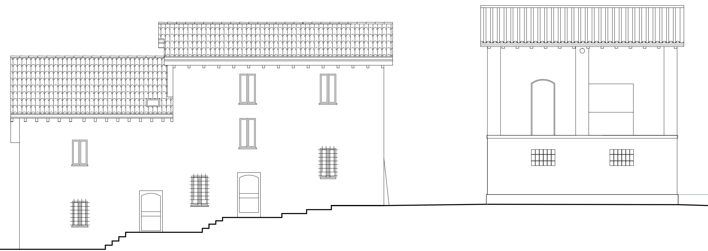
PROSPETTO OVEST
